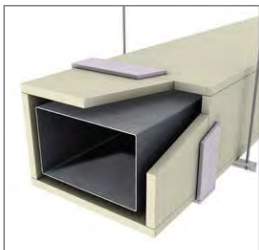
VZT potrubia s požiarную odolnosťou
